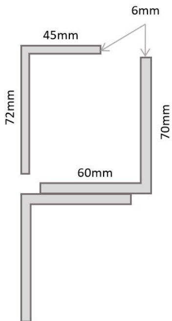
DIMENSIONS
